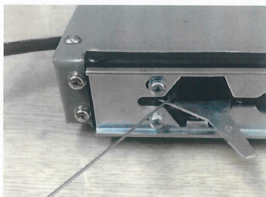
(b) 방진 시험 사진 ②
