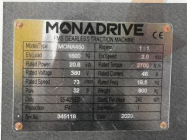
[사진 2] 구동기 제원 확인
