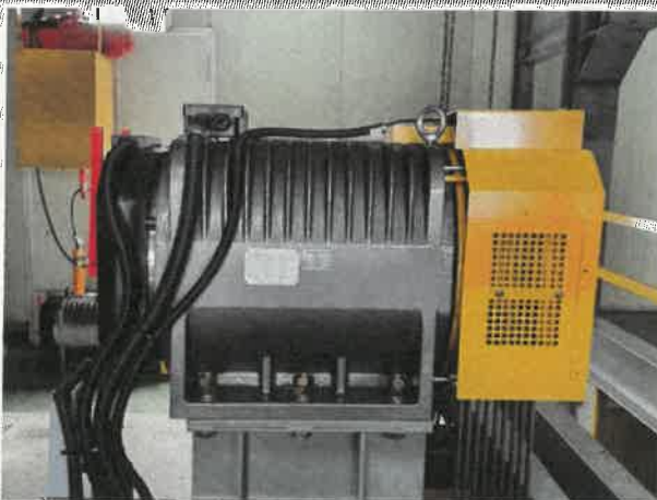
[사진 5] 동하중 시험 설치 및 작동상태 확인
