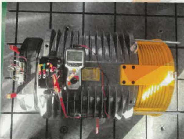
[사진 3] 전동기 절연저항 측정 시험
