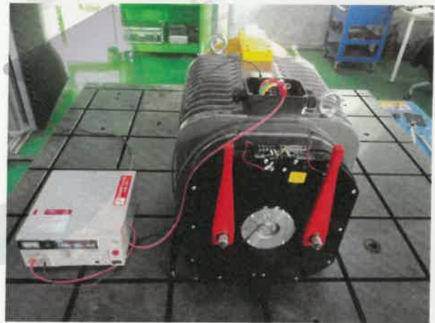
[사진 4] 무부하 운전중 소음 측정 시험
